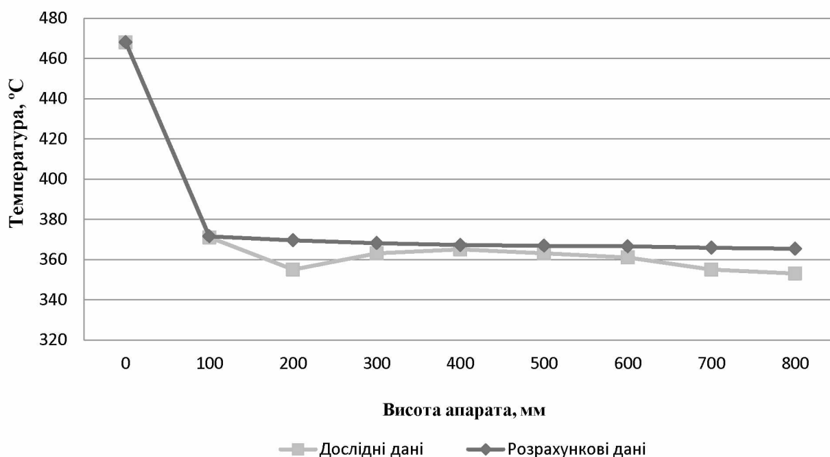
Рис. 5 – Зміна температури теплоносія по висоті апарата
