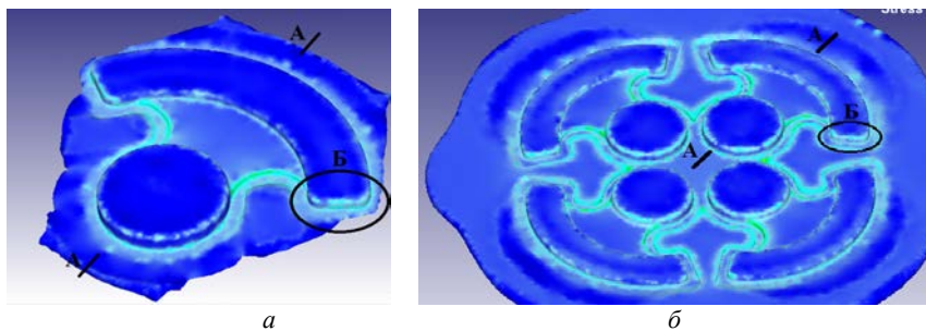
Рис. 6. Конечно-элементная модель отштампованной поковки и продольное сечение А-А и сечение Б-Б, в которых проводили анализ НДС: а – в обычном штампе; б - многоручная штамповка
