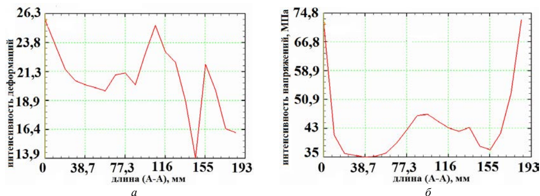
Рис. 10. Распределение интенсивности деформаций (а) и интенсивности напряжений (б) при многоштучной штамповке в сечении (А-А) после штамповки
