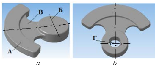
Рис. 1. Поковка «суппорт» (а) и деталь с отверстием (б):
