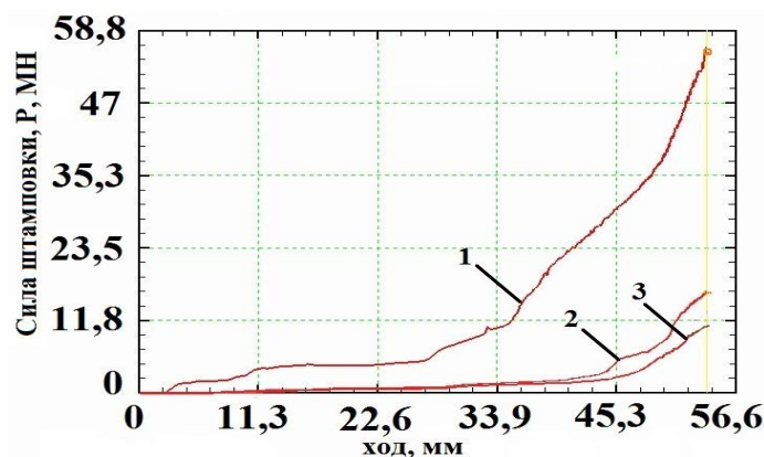
Рис. 12. График распределения силы необходимой для окончательно штамповки поковки «Суппорт»: 1 – многоштучная штамповка; 2 – штамповка без профилирования; 3 – штамповка с применением профилирования осадкой выпуклыми бойками
