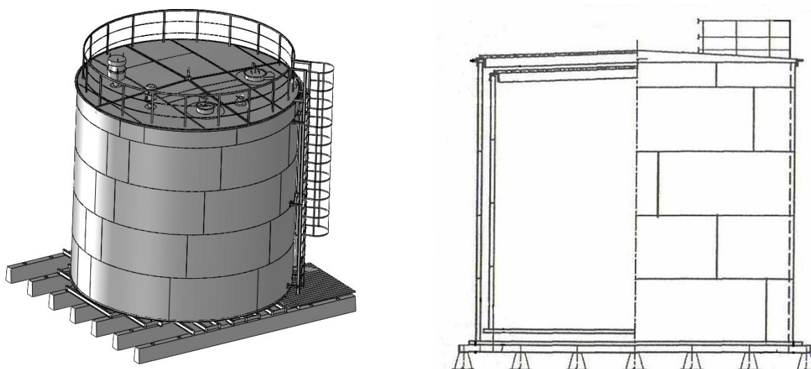
Рис. 1. Резервуар для зберігання дизельного палива, де: а) геометрична тривимірною модель; б) загальна схема конструкції
