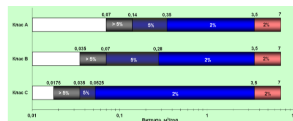
Рис. 3. Класи точності лічильників холодної води для DN25
