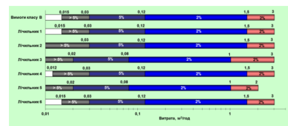
Рис. 11. Метрологічні характеристики поширених в Україні квартирних лічильників класу В
