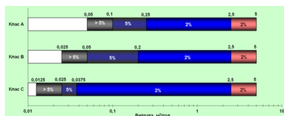
Рис. 2. Класи точності лічильників холодної води для DN20
