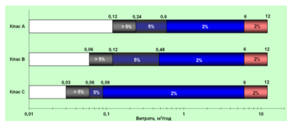
Рис. 4. Класи точності лічильників холодної води для DN32
