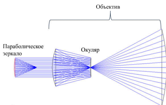
Рис. 4. Использование параболического зеркала – дополнительной фокусирующей системы в ППП Zemax
