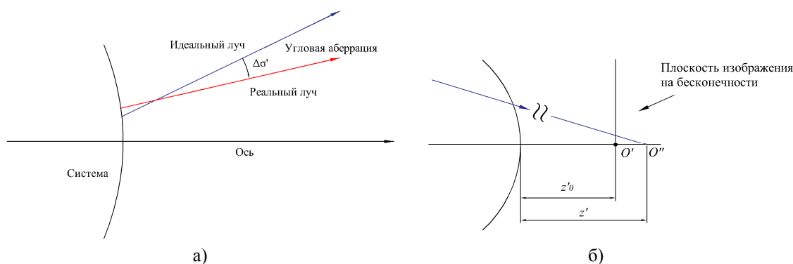
Рис 1. Представление геометрических aberrаций для удаленного изображения: а) в угловой мере; б) в линейной мере
