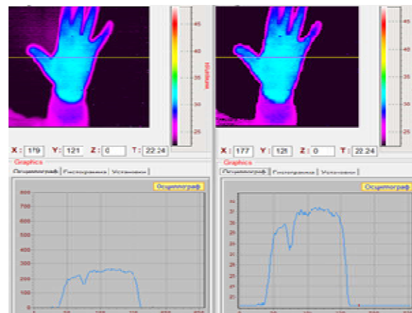
Рис. 4. Термограми зображень та осцилограми температурного профілю в відносних та реальних значеннях температури
