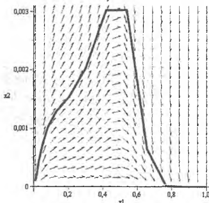
д) x_1(0)=0.01, x_2(0)=0.0001, t=0..120 , устойчивая точка (1;0)
