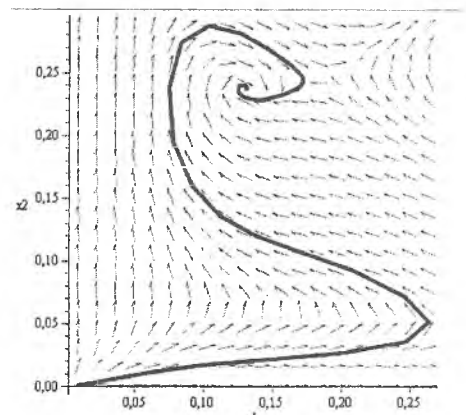
б) x_1(0)=0.009, x_2(0)=0.001, t=0..200 , устойчивая точка (0,1296;0.2380)
