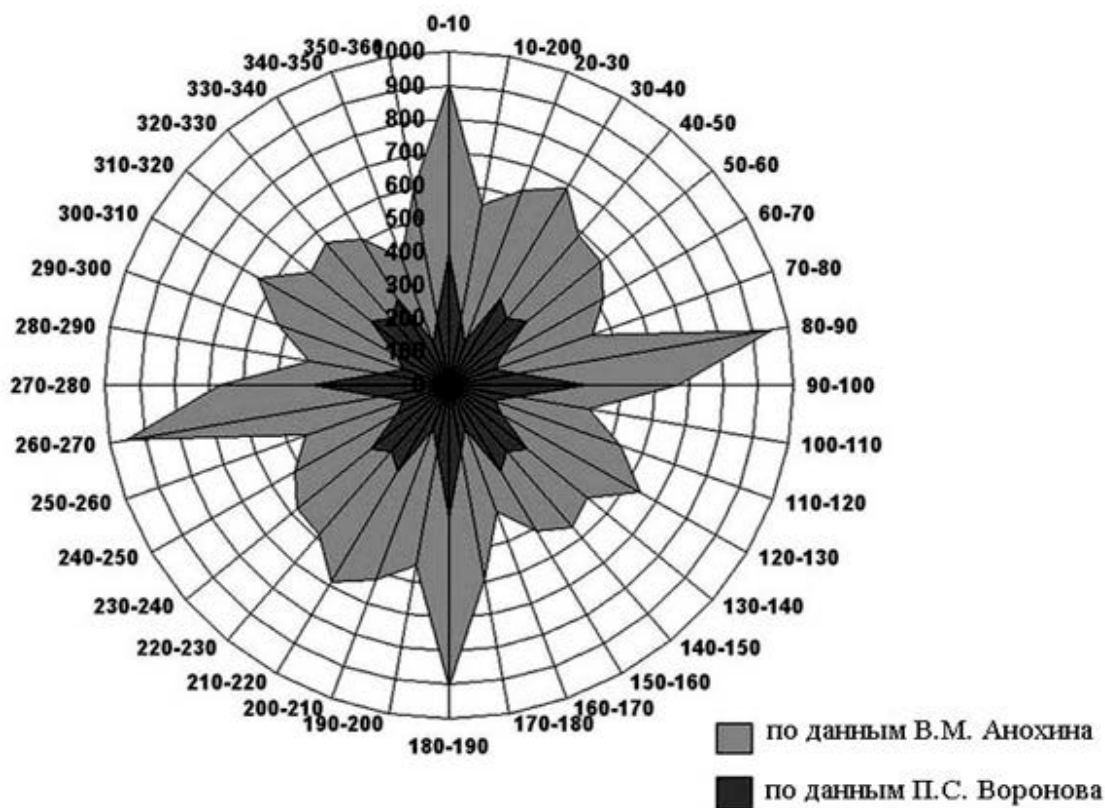
Рис. 1. Суммарная роза-диаграмма линейментов Земли, имеющих длину более 165 км. На круговой шкале – направления лимба, град., на радиальной – количество замеров.
