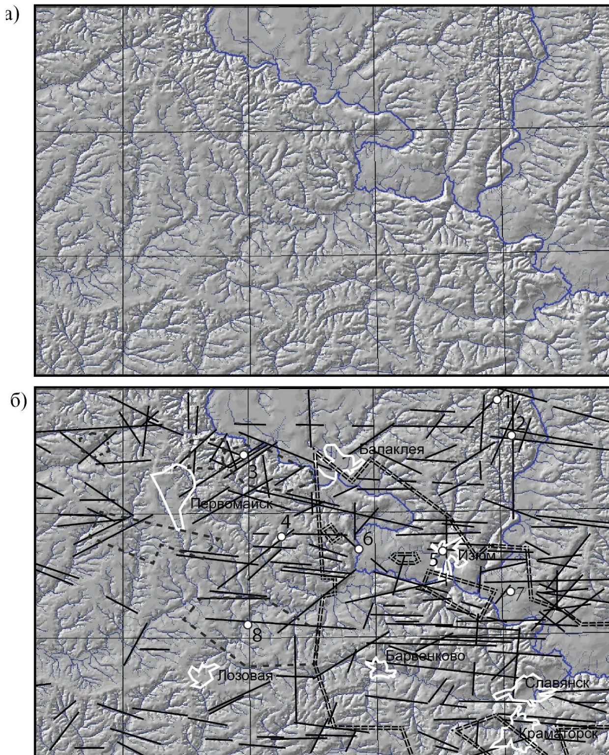
Рис. 3. Рельєф в районі середнього течення р.Северський Донець (часті Харківської і Донецької областей) - а) с лініями розривних порушень (прямі відрезки) і крупними родниками (кружки) – б).
