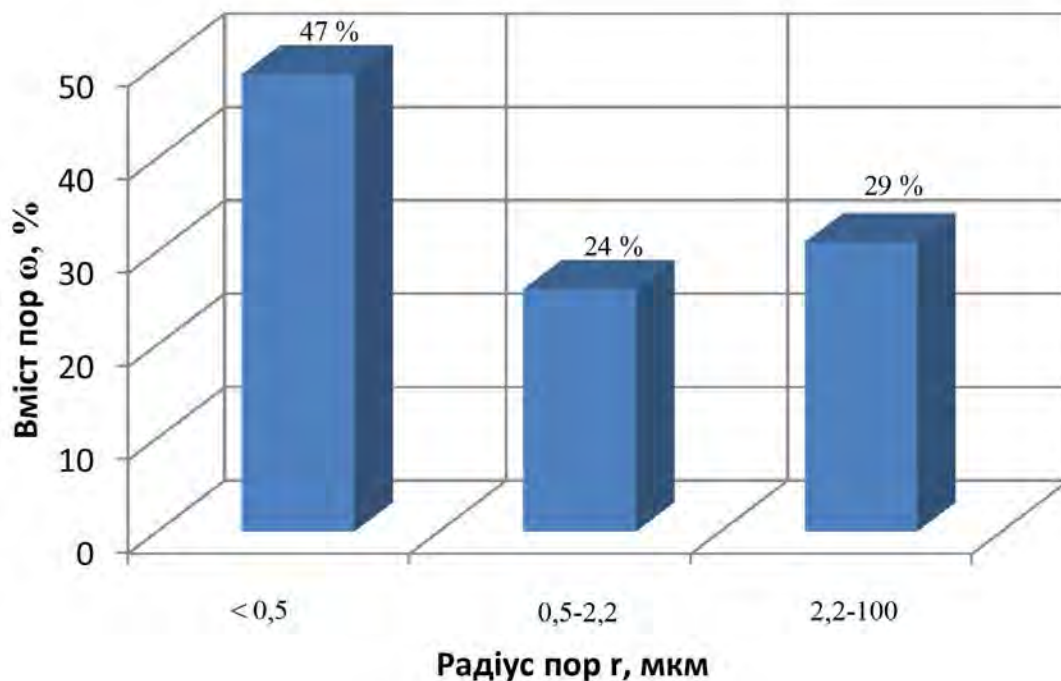
Рис. 5. Порометрична характеристика зразка GR-1, що має такі параметри: K_n = 21,9\% , K_{пр} = 6,9 мД, K_{пре} = 0,2 мД, K_{зв} = 46,6\%
