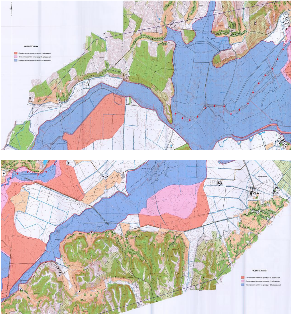
Рис.2. Зони затоплень території дослідження.
