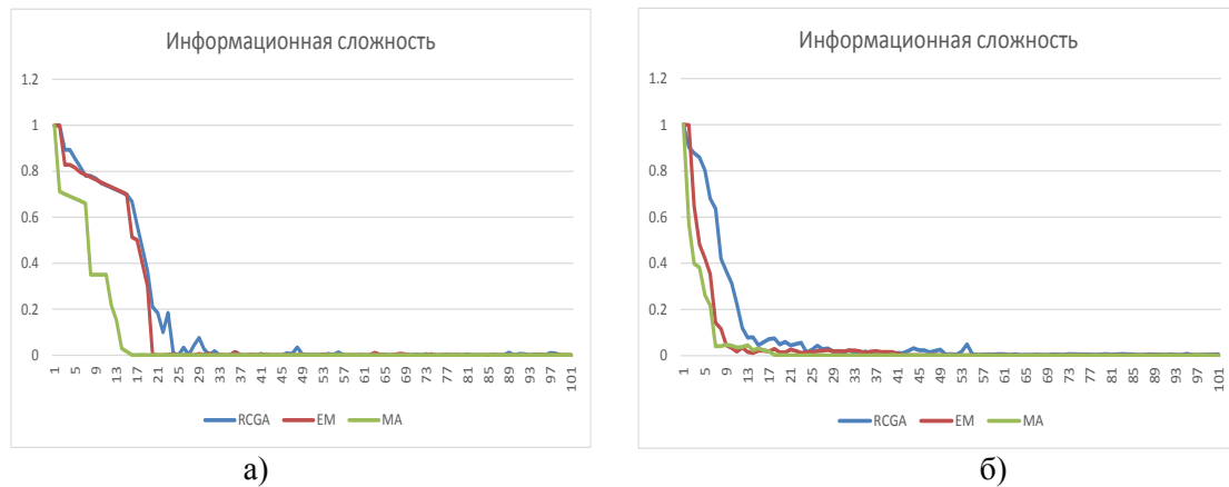
Рис. 1 – Результаты анализа сходимости предложенных вычислительных методов при решении задачи нахождения экстремума функции Розенброка в детерминированной (а) и стохастической (б) формулировках
