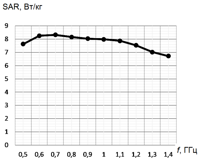
Рис. 4. Удельный коэффициент поглощения для всей капли как функция частоты.
