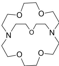
Рисунок 1. Структура криптана [2.2.1]
