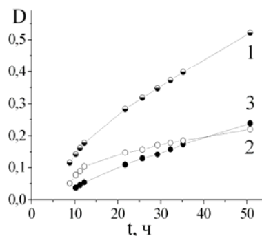
Рисунок 2. Зависимость оптической плотности (D) от времени (t) для частиц, образовавшихся в растворе АК в ДМСО: 1 - \text{AH}^- , 2 - \text{A}^{\cdot-} , 3 – ДКГК.
