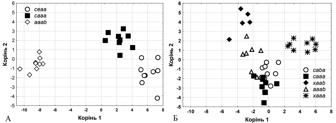
Рис. 1. Діаграма розсіяння в осях перших 2-х дискримінантних функцій (реплікації генотипів на генетичному фоні сорту Кооператорка (А) за алелями генів короткостебловості та Ppd-D1 : seaa – Rht8c , Rht-B1e , Rht-D1a , Ppd-D1a ; saaa – Rht8c , Rht-B1a , Rht-D1a , Ppd-D1a ; aaab – Rht8a , Rht-B1a , Rht-D1a , Ppd-D1b ; на генетичному фоні сорту Степняк (Б): за алелями caba – Rht8c , Rht-B1a , Rht-D1b , Ppd-D1a ; saaa – Rht8c , Rht-B1a , Rht-D1a , Ppd-D1a ; xaab – Rht8x , Rht-B1a , Rht-D1a , Ppd-D1b ; aaab – Rht8a , Rht-B1a , Rht-D1a , Ppd-D1b ; xaab – Rht8x , Rht-B1a , Rht-D1a , Ppd-D1a )
