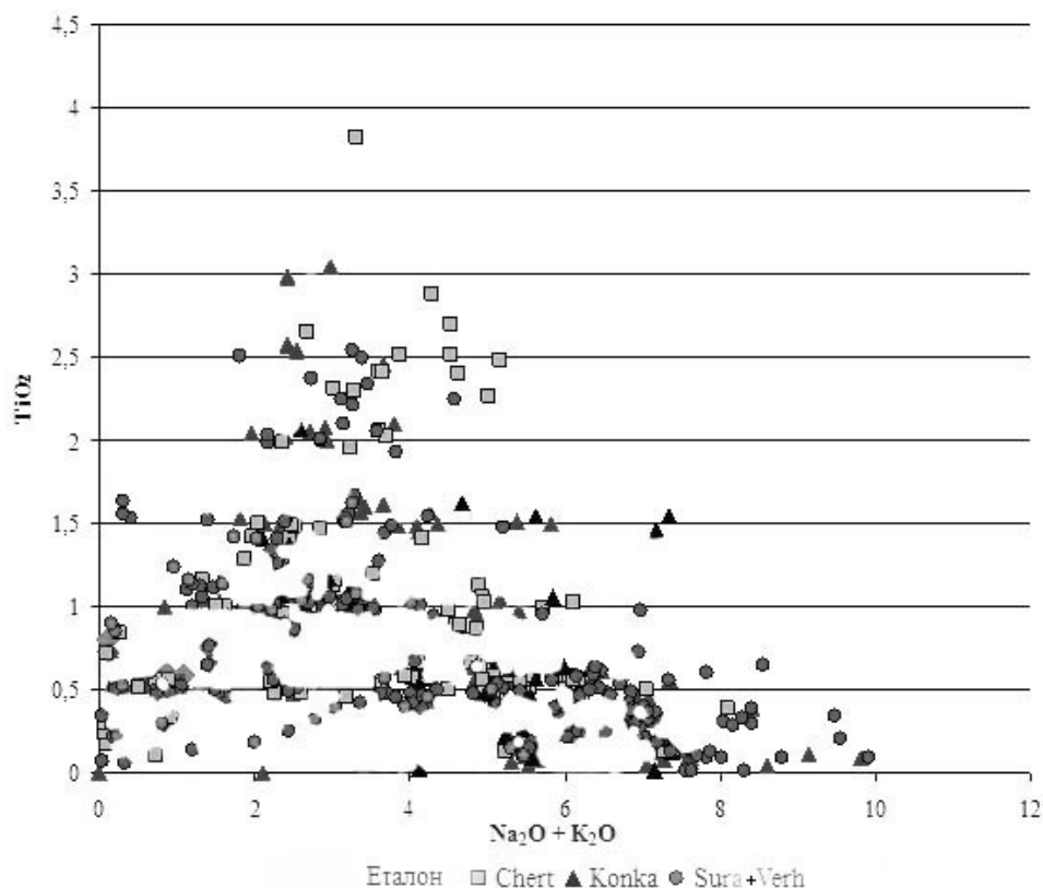
Рис. 5. Графік кореляції вмістів \text{TiO}_2 - (\text{Na}_2\text{O} + \text{K}_2\text{O}) в еталонному об'єкті та окремих областях розвитку коматїтів Українського щита, структури: Chert – Чортомликська, Konka – Конкська, Sura – Сурська, Verh – Верхівцевська.
