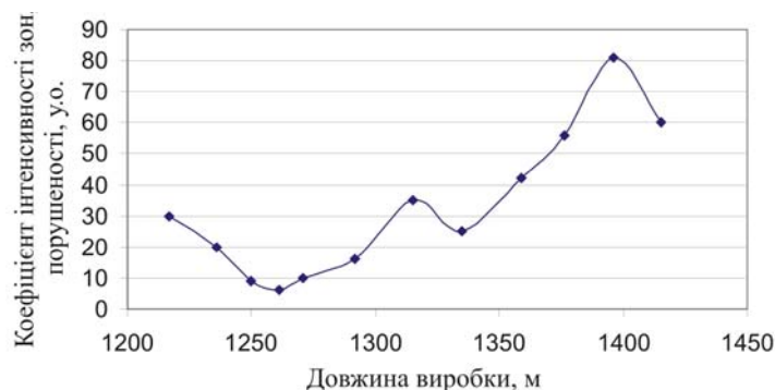
Рис. 2. Графік зміни K_{\text{зп}} в області розвитку Ветковського насуву по 17-му західному конвеєрному штреку пласта m_3 .
