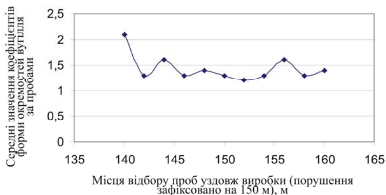
Рис. 4. Графік зміни середніх значень Кф окремоостей вугілля за пробами з шахти ім. Л. І. Лутугіна.
