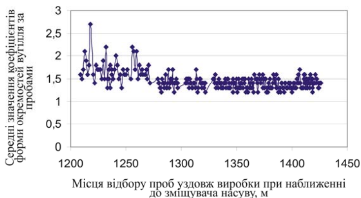
Рис. 3. Графік зміни середніх значень K_{ф} окремої вугілля за пробами з шахти ім. О. Ф. Засядька.
