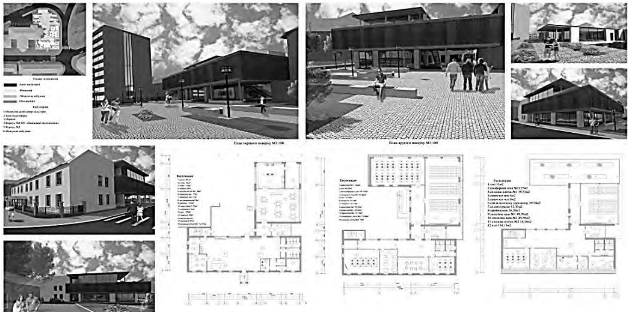
Рис. 8. Архітектурне вирішення Міжвузівського центру культури на вул. С. Бандери у м. Львові
