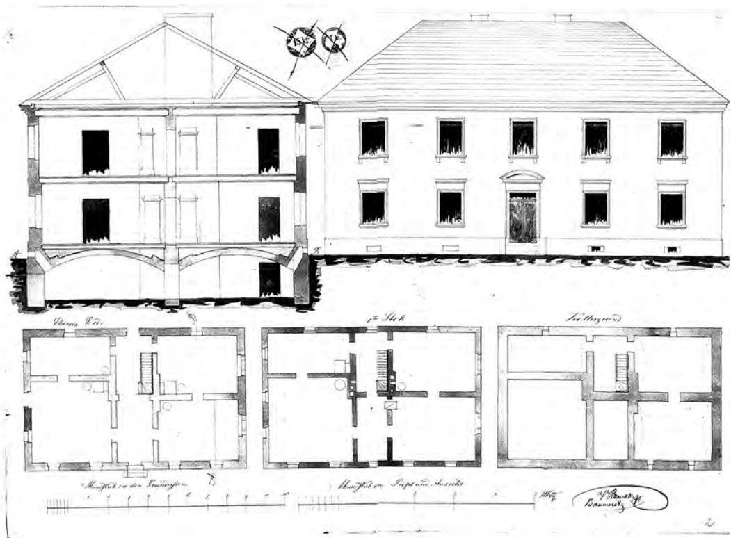
Рис. 6. Проект будинку № 2 на вулиці Городоцькій. Архівне креслення[20]
