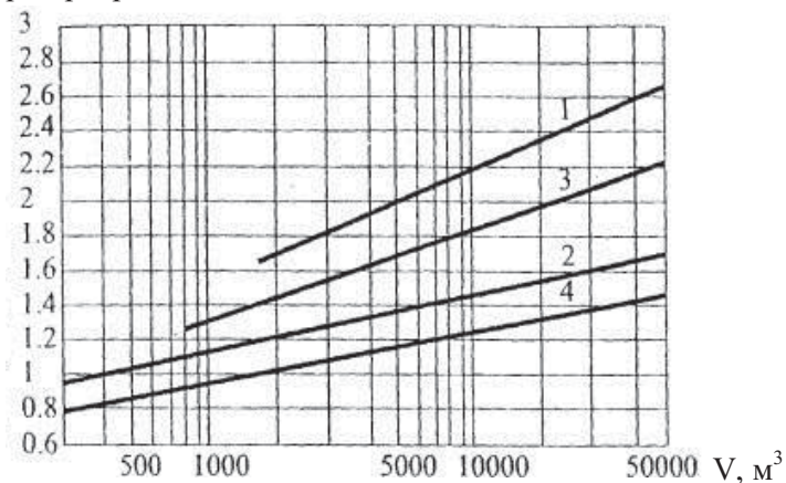
Рис. 2. Залежність оптимальних значень часу реверберації від об'єму приміщення за частоти 512 (500) Гц:
