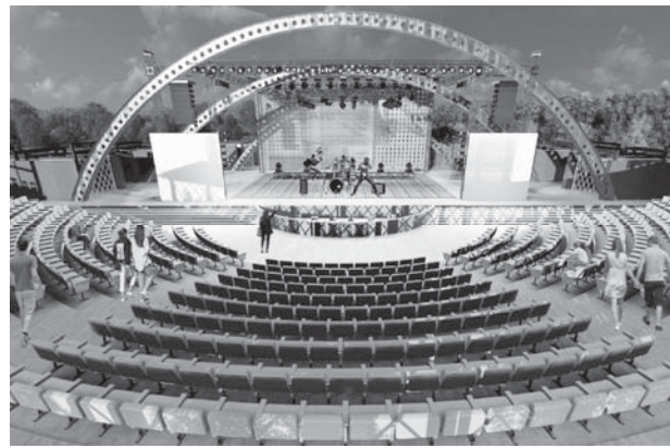
Рис. 4. Бакалаврська кваліфікаційна робота під назвою: “Дизайн архітектури ландшафтного театру в садибі Тобілевичів під м. Кропивницьким”. Виконала в 2017 р. студентка І. Забігайло під керівництвом д-ра арх., проф. В. І. Проскуракова, асист. І. В. Гуменник
