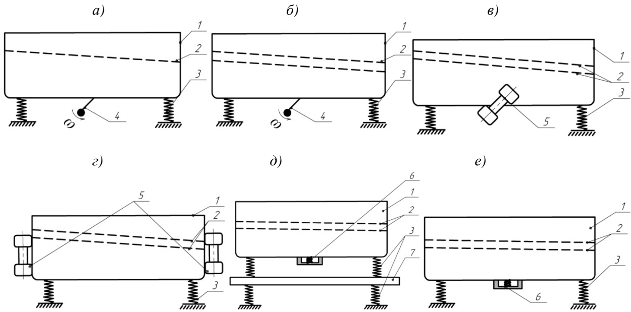
Рис. 3. Принципові схеми вібраційних сепараторів: 1 – корпус вібросепаратора; 2 – сита; 3 – пружини; 4 – дебаланс; 5 – мотор-вібратор; 6 – електромагнітний вібробудник; 7 – рама
