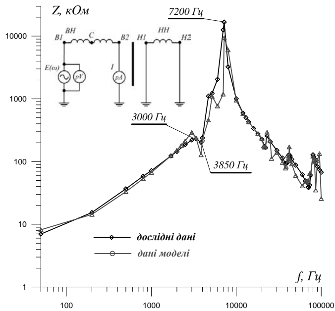
Рис. 4. Схема та частотні характеристики досліду КЗ НОМ-10
