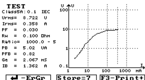
Рис. 2. VA-характеристики
