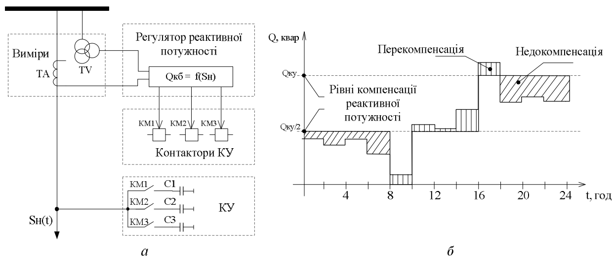
Рис. 2. Автоматичне регулювання реактивної потужності для вузла навантаження: а – принципова схема; б – ефект роботи регулятора реактивної потужності на графіку навантаження вузла ЕПС
