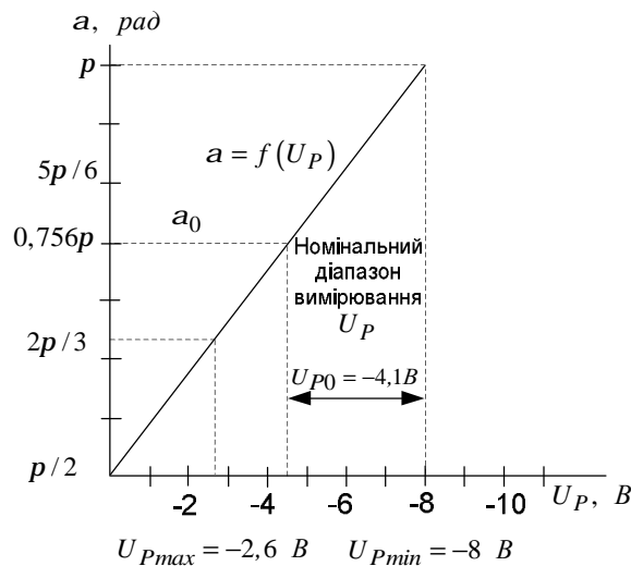
Рис. 4. Прогідна характеристика СІФК СТК
