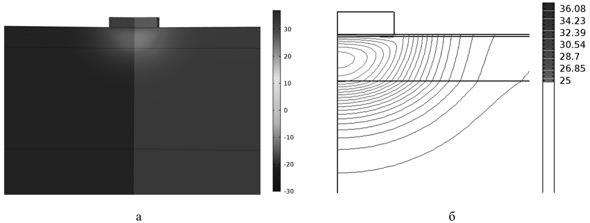
Рис. 1. Розподіл температури (а) та ізотермічних поверхонь (б) в об'ємі шкіри, на поверхні якої розміщено робочий інструмент, за температури T = +30^{\circ}\text{C} у момент часу t = 30\text{ с}
