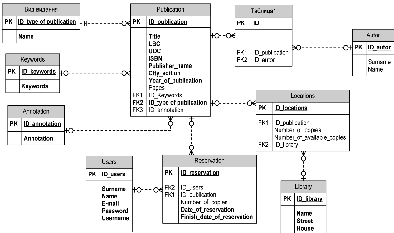
Рис. 7. Діаграма “сутність-зв’язок”
