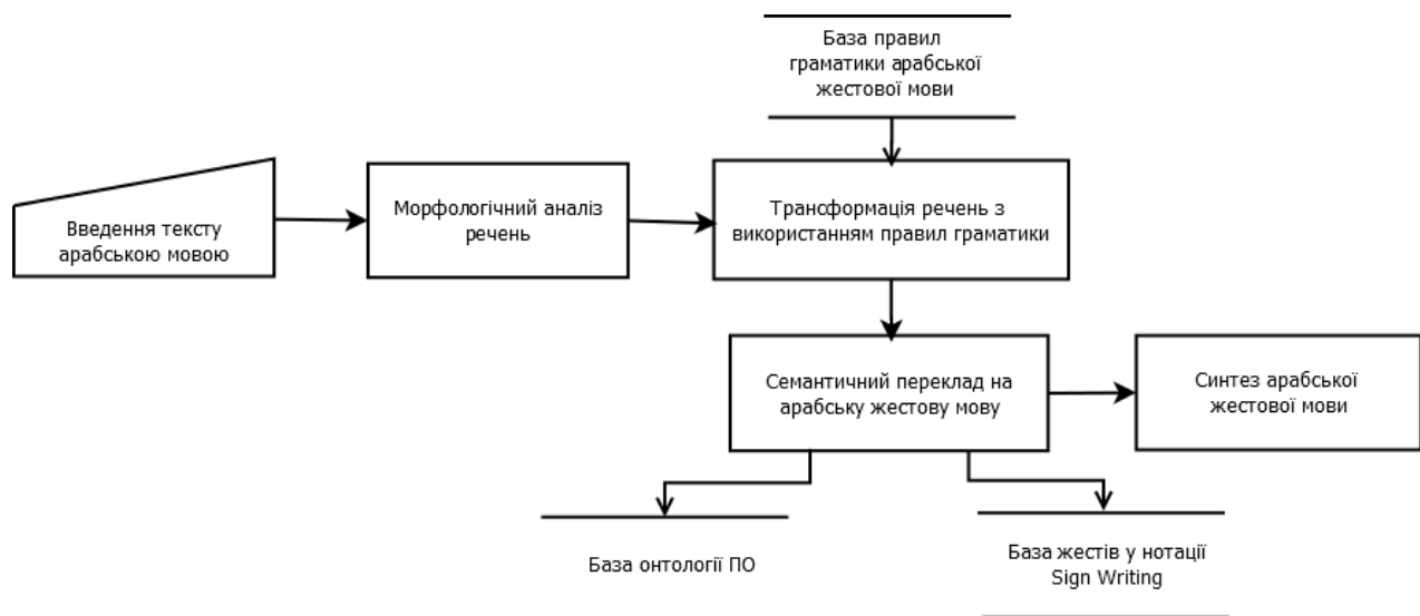
Рис. 4. Схема системи перекладу на арабську жестову мову з використанням онтології
