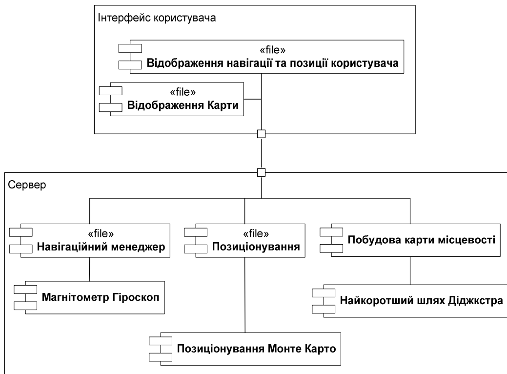
Рис. 8. Архітектура системи GROPING [36]
