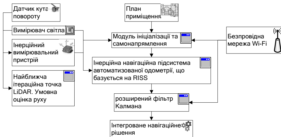
Рис. 6. Архітектура IINSGV
