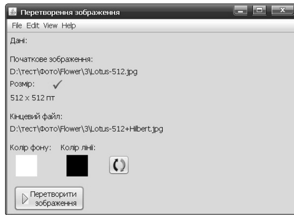
Рис. 14. Інтерфейс програми
