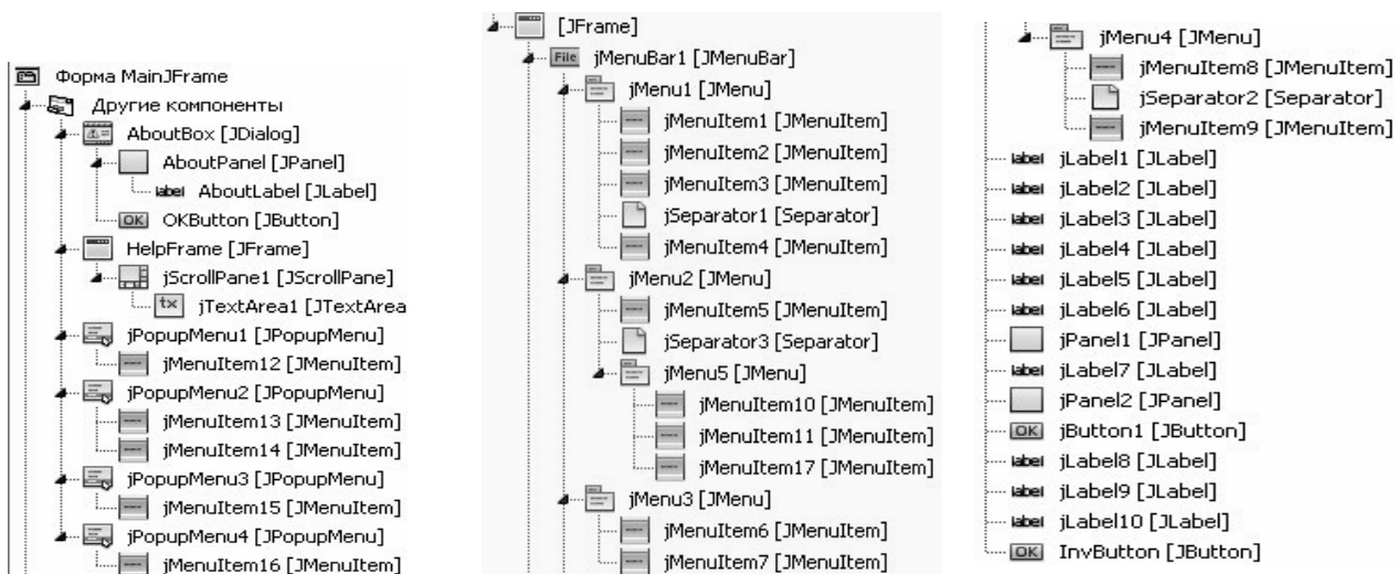
Рис. 7. Компоненти ПЗ
