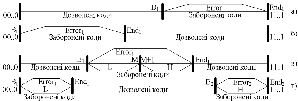
Рис. 3. Дозволені і заборонені коди розрядів елементів полів Галуа GF(d^m)
