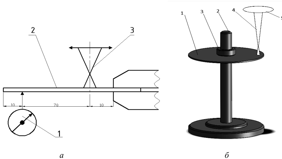
Рис. 1. Схема проведення експерименту: а – пластин (1 – індикатор переміщення, 2 – зразок, 3 – лазерний промінь); б – дисків (1 – зразок, 2 – стійка, 3 – фіксатор, 4 – лазерний промінь, 5 – лінза)
