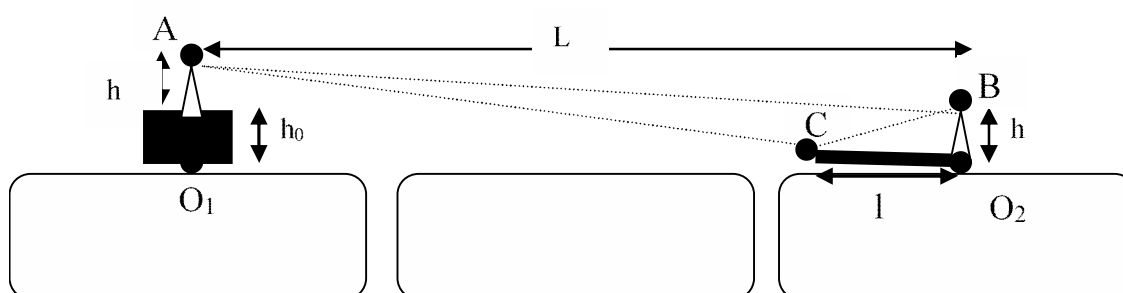
Рис. 7. Линейные размеры отражающей системы
