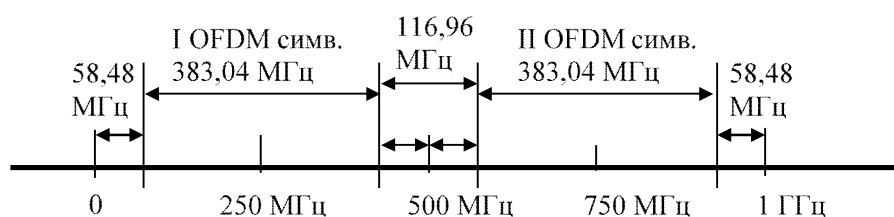
Рис. 2. Размещение OFDM символов в полосе 1 ГГц
