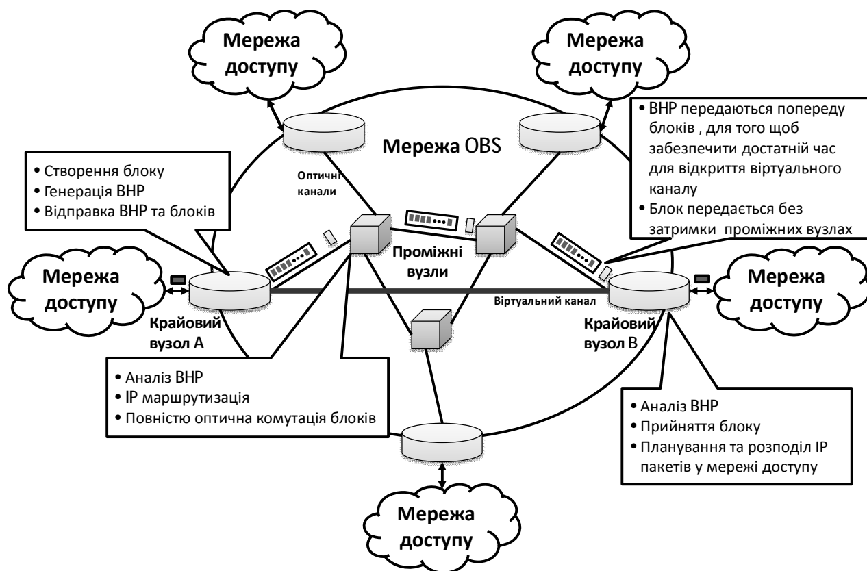
Рис. 1. Процес передавання даних у мережі з оптичною комутацією блоків
