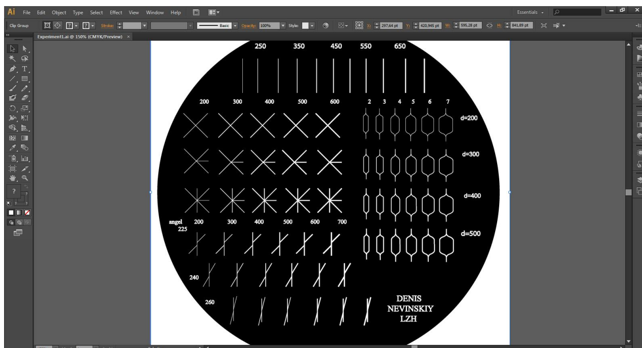
Рис. 2. Робоче вікно з дизайном хвилюводів різних конфігурацій
