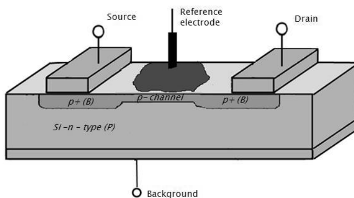
Fig. 1. ISFET structure
