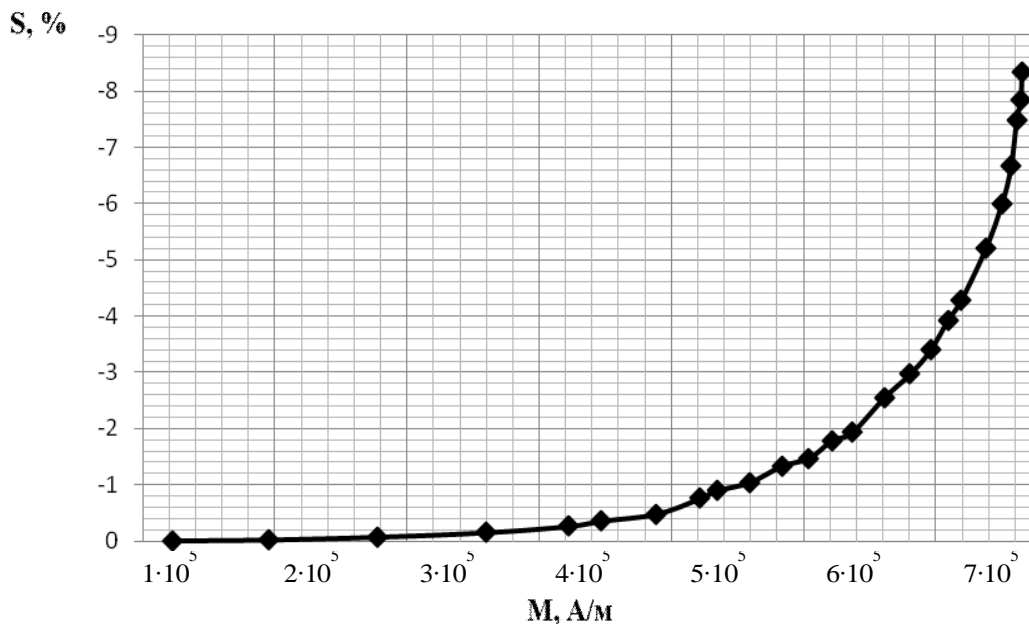
Рис. 3. Параболічна залежність коефіцієнта від'ємного магнітоопору від намагніченості в ниткоподібних мікрочисталах Si_{1-x}B_x , T=4,2 K
