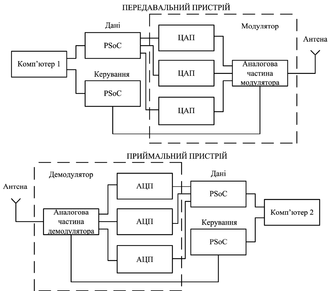
Рис. 4. Структурна схема вискоефективної системи, основаної на використанні АМБС
