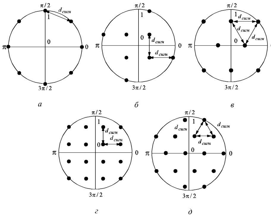
Рис. 1. Сигнальні сузір'я: а – 8-ФМ-сигналу; б – 8-КАМ-сигналу; в – 8-АМБС-сигналу (три складові) зі зсувами; г – 16-КАМ-сигналу; д – 16-АМБС-сигналу (три складові) зі зсувами
