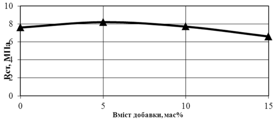
Рис. 3. Вплив добавки цеоліту на міцність гіпсового в'язучого через 2 години
