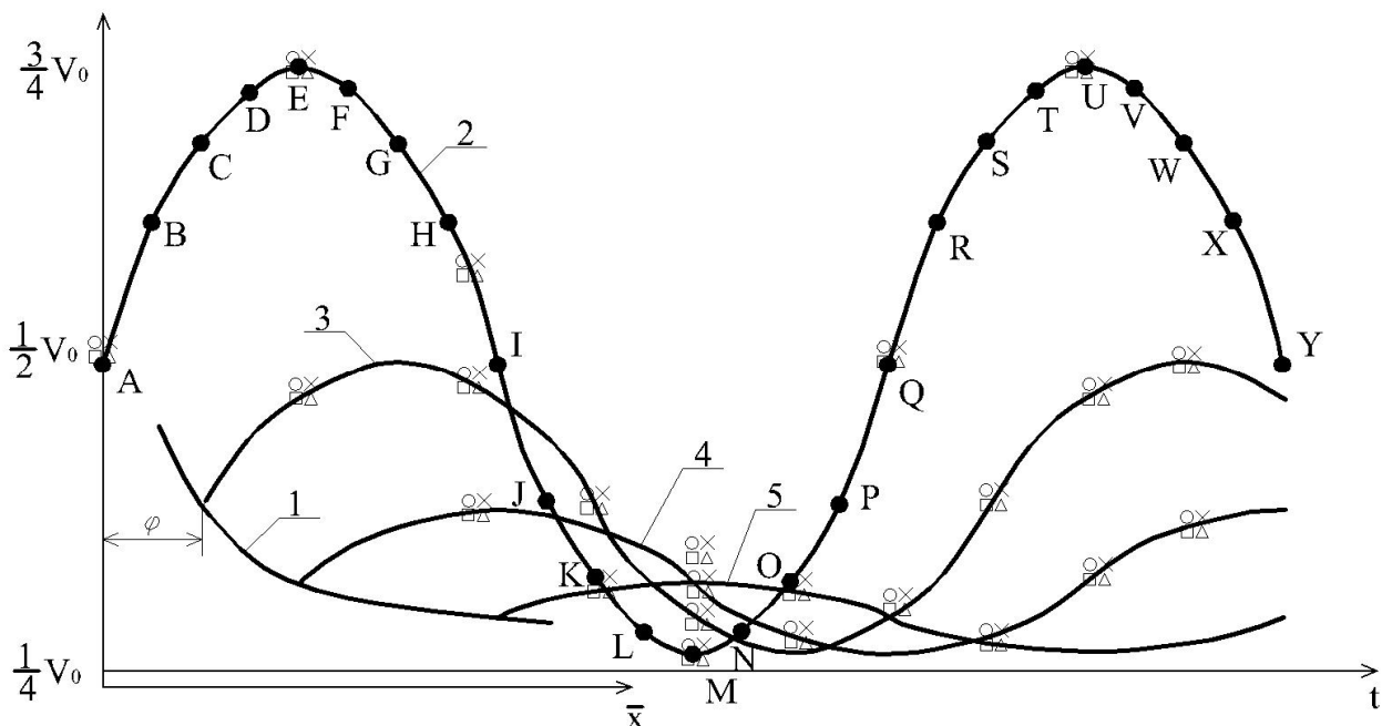
Рис. 1. Результати досліджень: 1 – залежність швидкості від координати при стаціонарному режимі; 2, 3, 4, 5 – залежності швидкості від часу при різних координатах (нестаціонарний режим)
