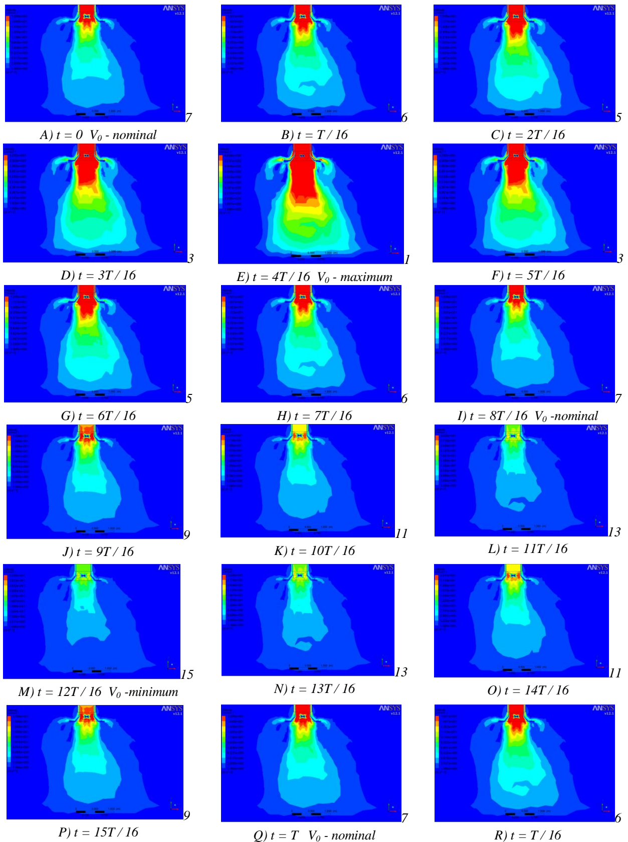
Рис. 3. Етюри швидкостей припливного повітряного потоку в січєнні повітророзподільника при подачі повітря закрученими і настільними струминами при куті нахилу закручувальних пластин 60^\circ і при проміжку часу t = T/16 (1 хв) (модель Спаларта–Алмараса)
