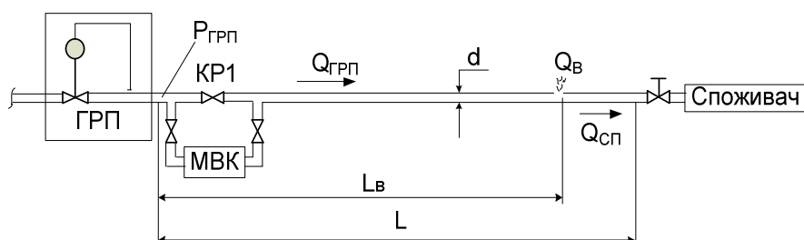
Рис. 1. Спрощена схема ділянки газорозподільної мережі із виявленими витокami
