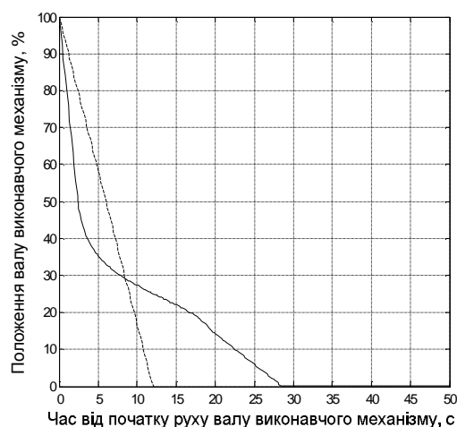
Рис. 5. Переміщення валу виконавчого механізму за частоти живлення двигуна 50 Гц (---) та зміни частоти живлення двигуна відповідно до положення заслінки (—)
