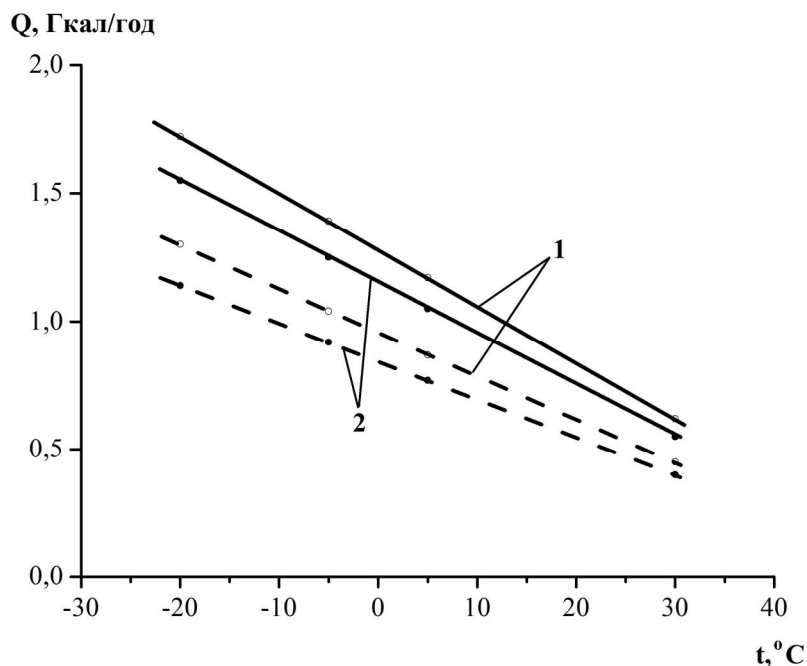
Рис. 1. Залежність втрати тепла котлом ПТВМ-180 від температури навколишнього повітря: 1 – температура мережевої води на вході у котел 73 °С; 2 – температура мережевої води на вході у котел 64 °С; ——— - шибер за котлом відкритий; - - - - - шибер за котлом закритий
