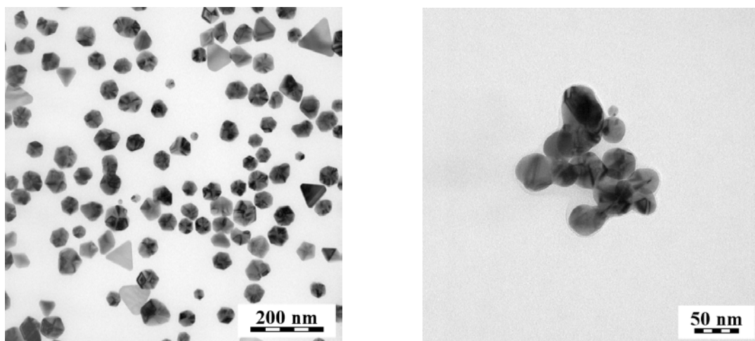
Рис. 3. ТЕМ фотографії колоїду з наночастинками срібла, отримані з аргентуму нітрату (а) і аргентуму ацетату (б) у розчині ПВП: [AgNO_3]:[PVP]:[H_2O] = 1:10:10 мас.ч., M_{PVP} = 10^4 , T = 348 К, тривалість реакції – 1 год
