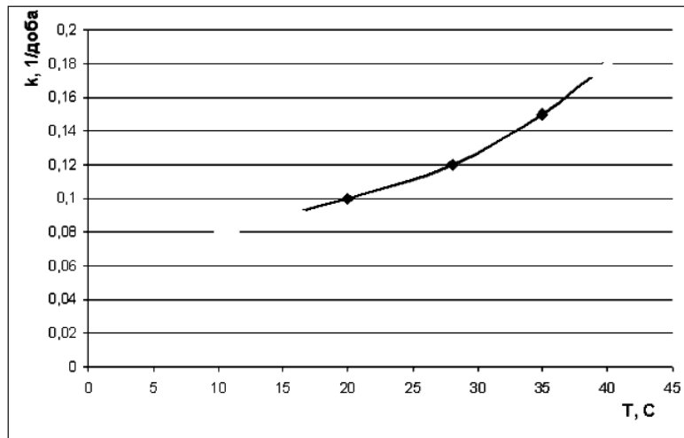
Рис. 3. Залежність коефіцієнта приросту – k мікробіодоростей від температури – T^{\circ}C
