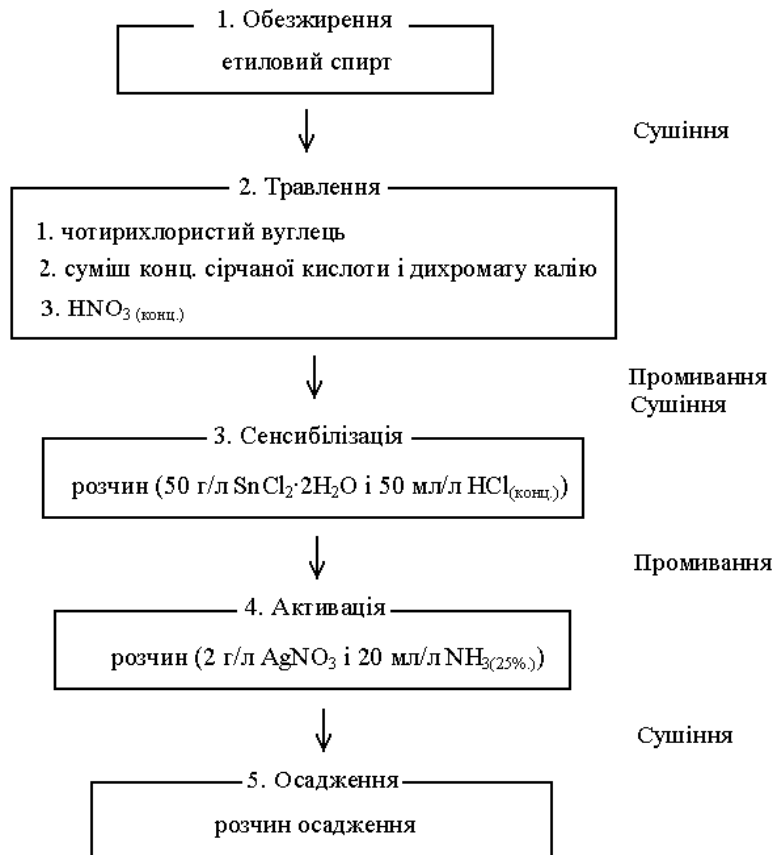
Рис. 1. Схема металізації полівінілхлоридного пластикату за класичною технологією
