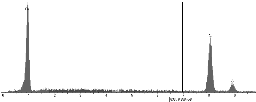
Рис. 8. Спектр характерного рентгенівського випромінювання мідного полівінілхлоридного пластикату
