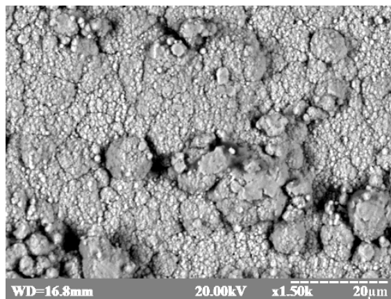
Рис. 7. Мікрофотографії поверхні мідного ПВХ пластикату одержані у режимі контрасту по середньому атомному номеру
