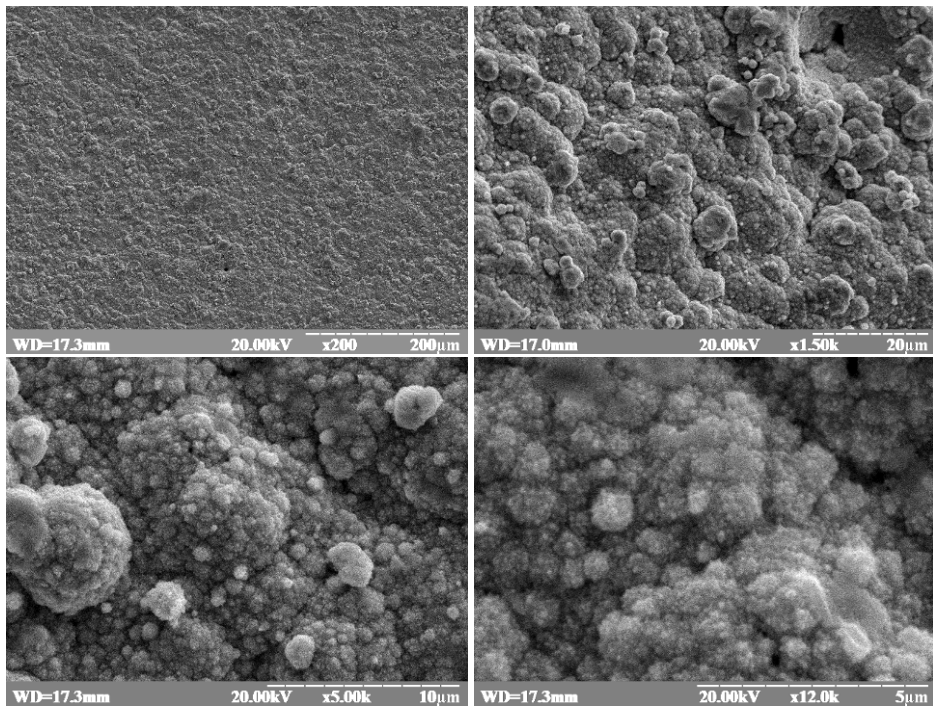
Рис. 6. Мікрофотографії поверхні мідного ПВХ пластикату
