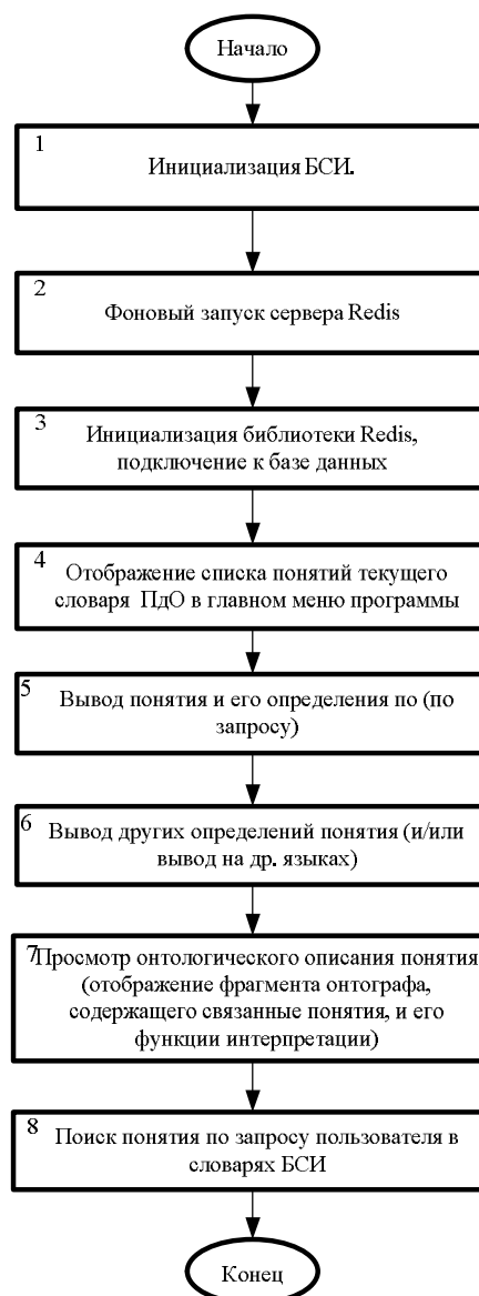
Рис. 8. Обобщенный алгоритм работы модуля БСИ для работы в пользовательском режиме
