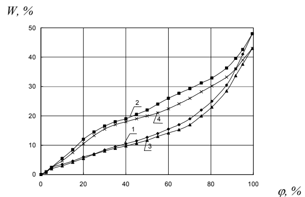
Рис. 1. Ізотерми сорбції-десорбції шкіри хромового методу дублення без покриття (криві 1, 2); шкіри хромового методу дублення з нітроемulsionним покриттям (3, 4): 1, 3 – ізотерма сорбції; 2, 4 – ізотерма десорбції
