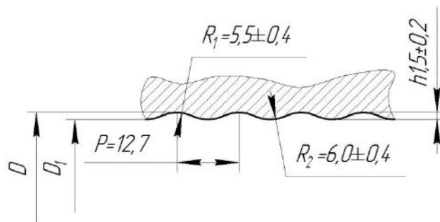
Рисунок 1 – Изображение круглой резьбы
