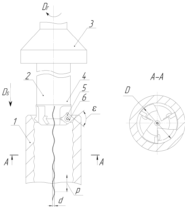
Рисунок 2 – Схема формообразования круглой резьбы
